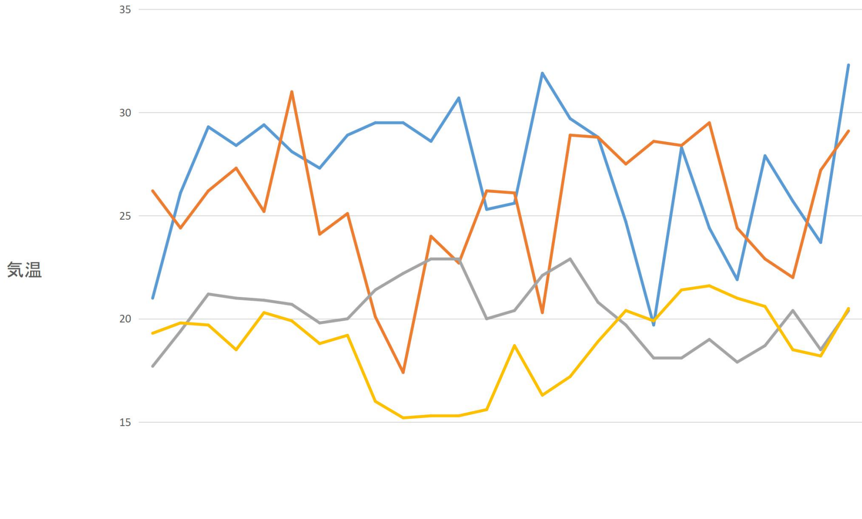
横浜の気温比較(2020年6月vs2019年6月)
